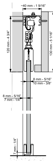
ALZADO KT GLAS 80
