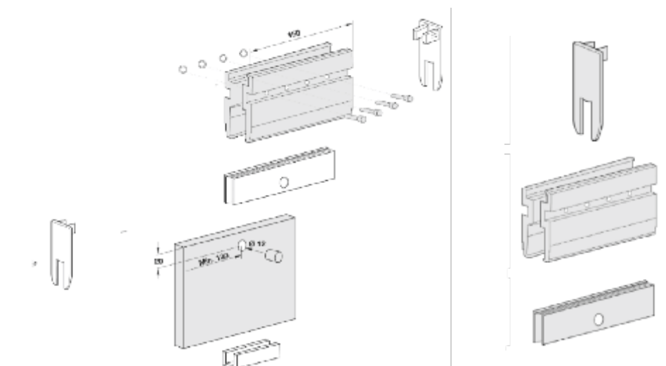
Brida para clipar izquierda
