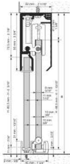
ALZADO ROLLGLAS 60-90 EXPERT
