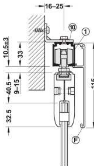
Montaje mural con escuadra de montaje y pantalla para clipar 115 mm
