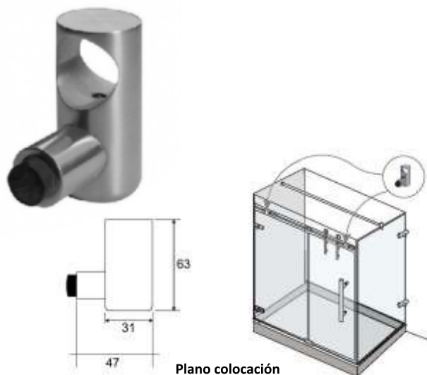
Plano colocación
