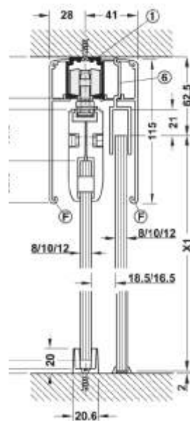
Montaje a techo con carril de deslizamiento y pantalla para clipar 115 mm incluida pieza fija para bases de madera, selado en húmedo
