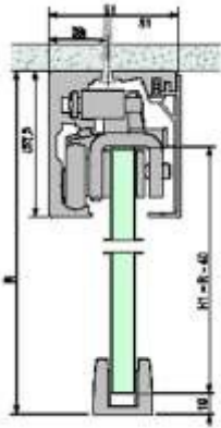
Detalle techo
