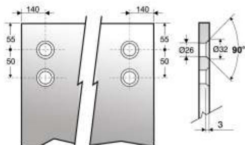
Muesca
