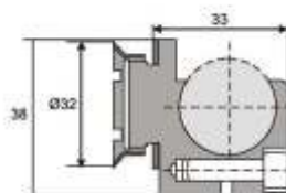
Plano colocación
