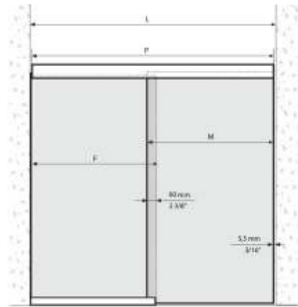
Pin L-5 mm (máx. 3 m) Pin L-3/16\" (máx. 9' 10.1/8\")
