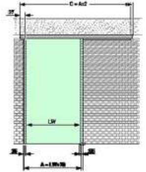
Detalle 1 hoja
